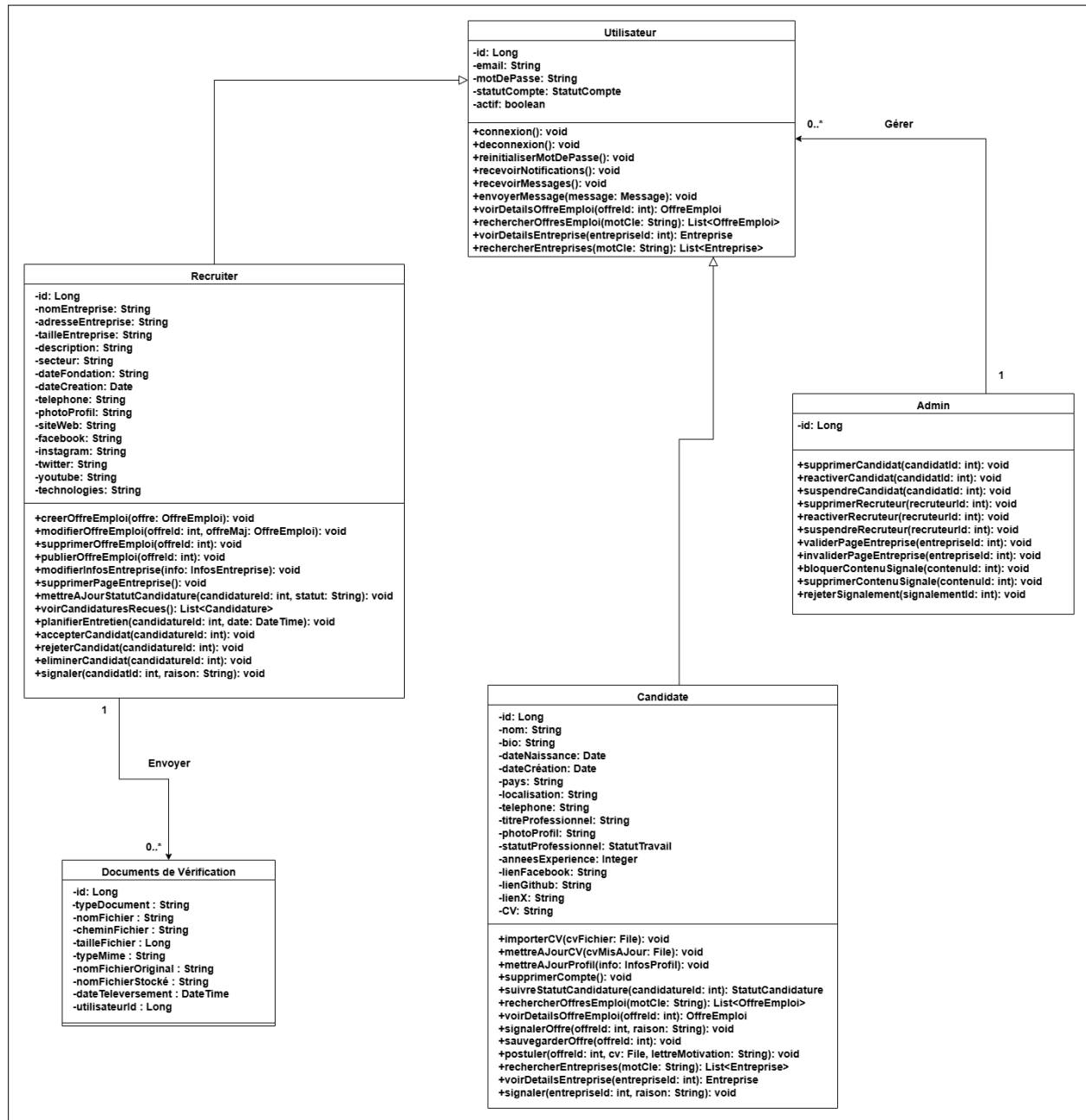
Figure 62 - Diagramme de classe du sprint 1
